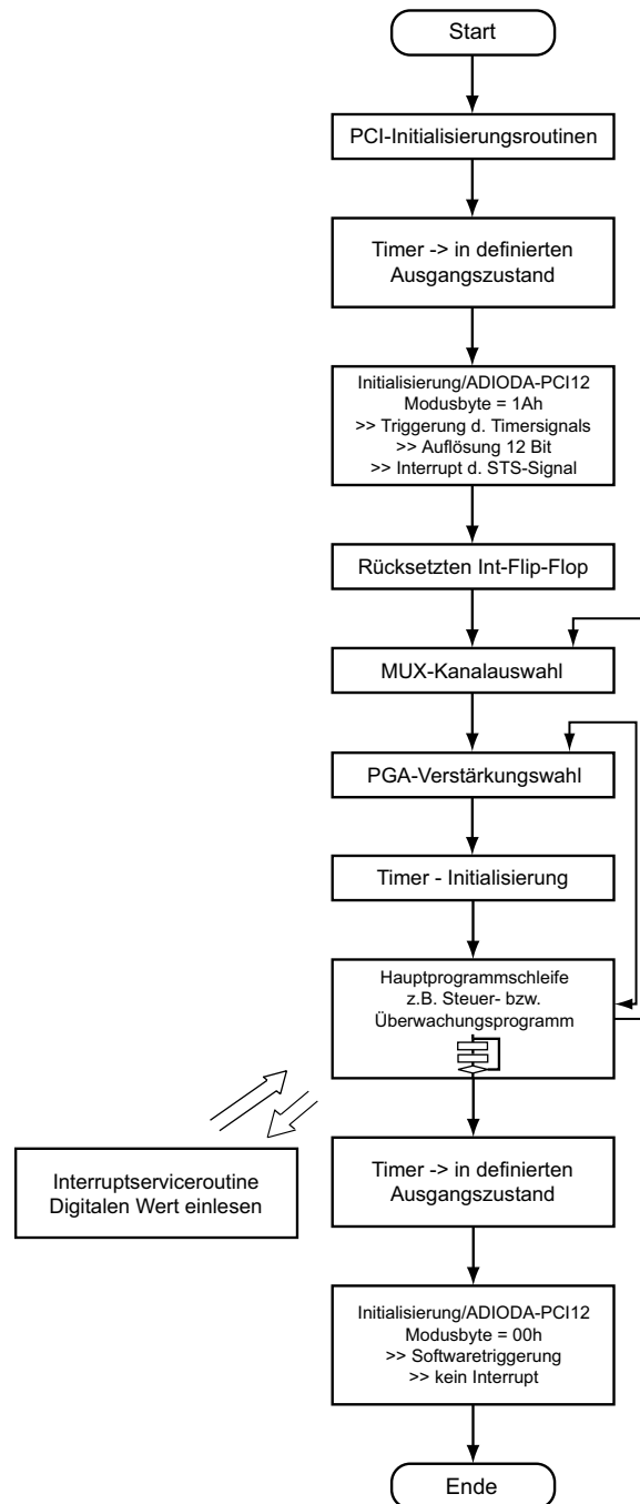
Ablaufdiagramm/ 12-Bit-Wandlung (Timer-Auslösung/STS-Interrupt)
