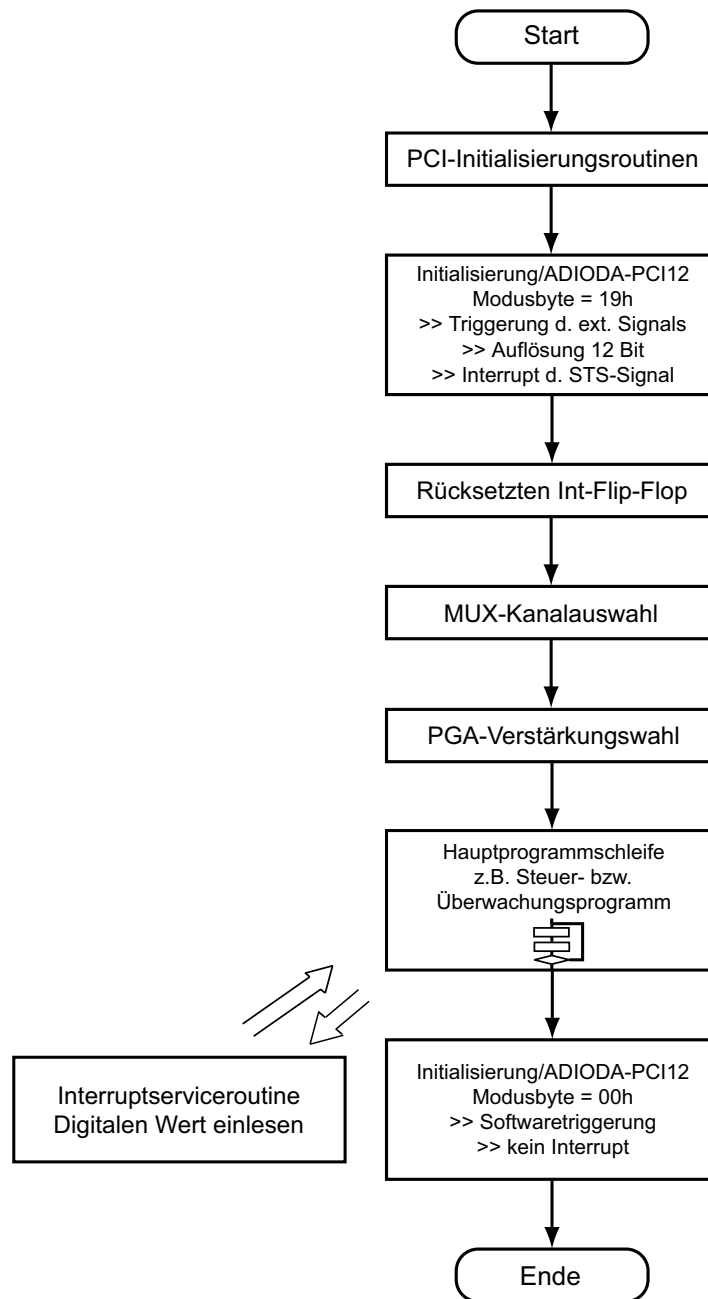
Ablaufdiagramm/12-Bit-Wandlung (Externe Triggerung/STS-Interrupt)
