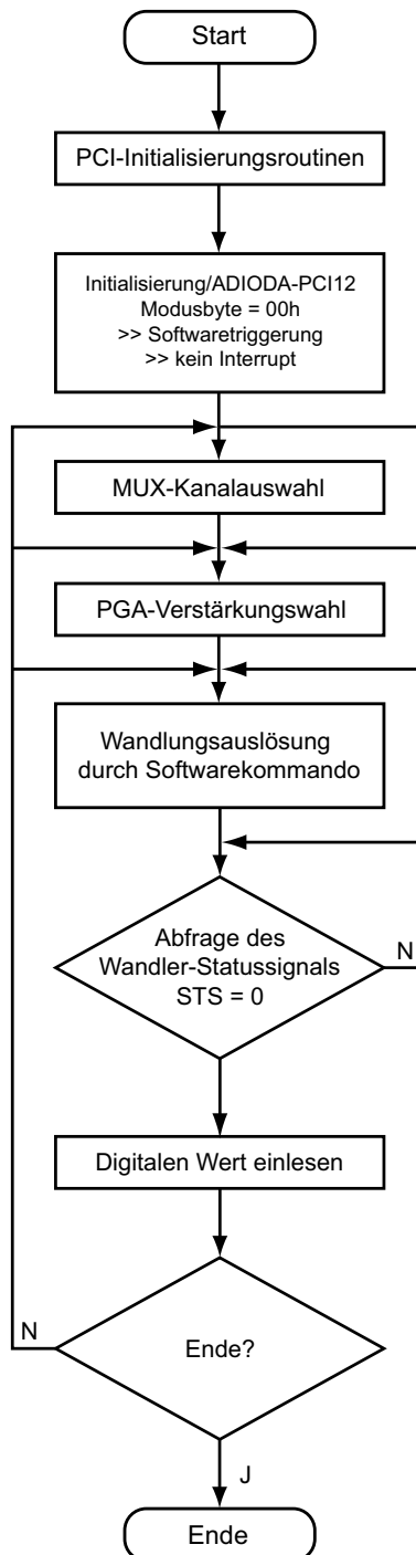
Ablaufdiagramm/ 12-Bit-Wandlung (Softwaretriggerung/STS-Polling)
