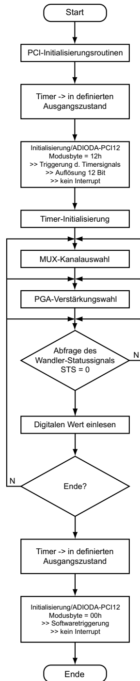
Ablaufdiagramm/ 12-Bit-Wandlung (Timer-Auslösung/STS-Polling)
